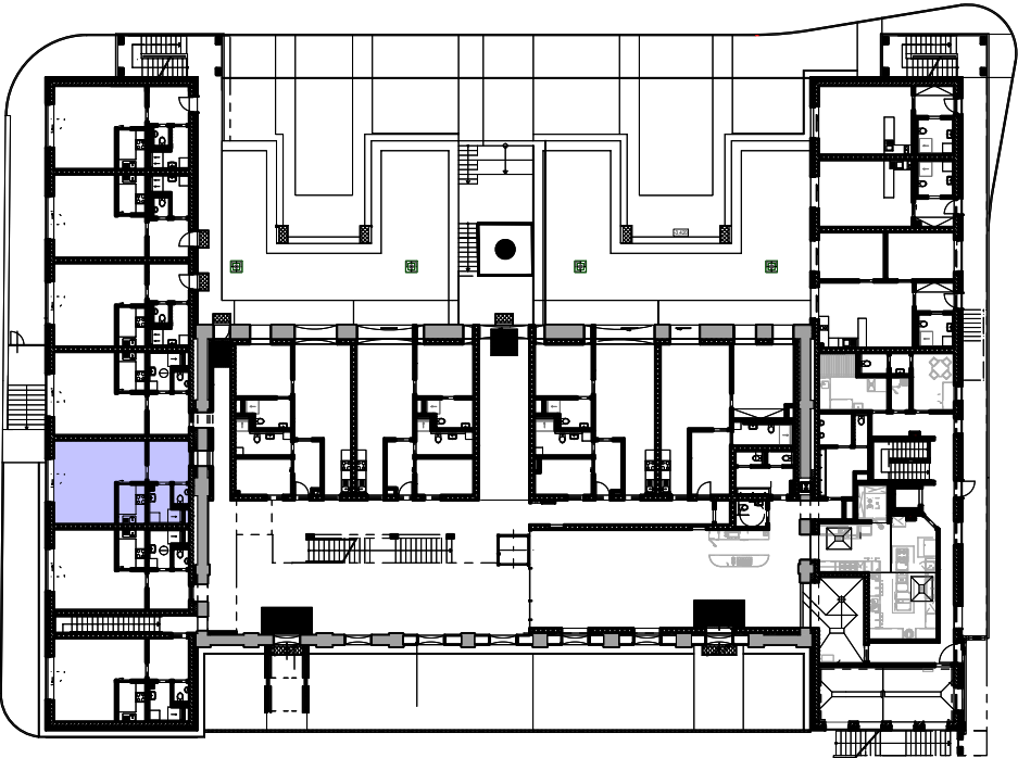
Schéma půdorys
